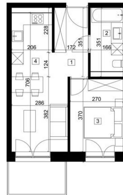
PLAN MIESZKANIA 1:100
