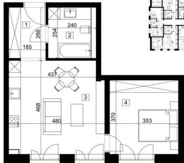
PLAN MIESZKANIA 1:100
